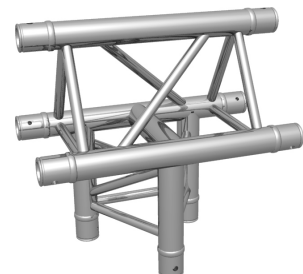
F33 3-Wege T-Stück vertikal F33 3-way T-piece vertical
