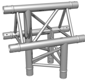
F33 3-Wege T-Stück horizontal F33 3-way T-piece horizontal
