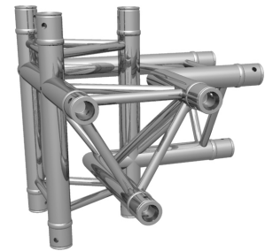
F33 4-Wege Ecke unten/rechts F33 4-way corner bottom/right
