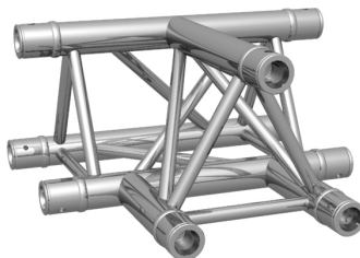
F33 3-Wege T-Stück horizontal F33 3-way T-piece horizontal
