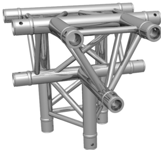
F33 4-Wege T-Stück unten F33 4-way T-piece bottom
