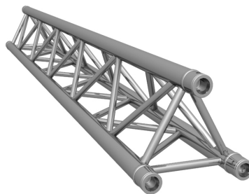
F33 250 cm F33 250 cm
