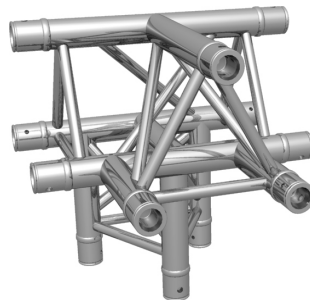
F33 4-Wege T-Stück oben F33 4-way T-piece top
