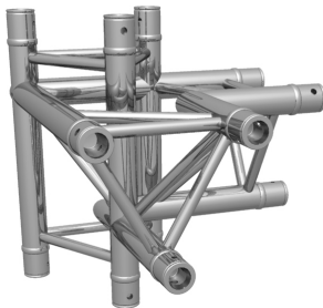
F33 4-Wege Ecke unten/links F33 4-way corner bottom/left
