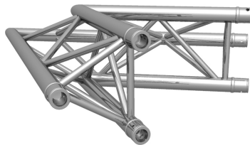
F33 2-Wege Ecke 60° außen F33 2-way corner 60° outside
