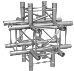
F24 6-Wege Ecke F24 6-way corner
