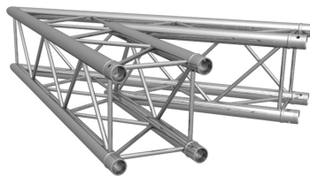
F24 2-Wege Ecke 45° F24 2-way corner 45°
