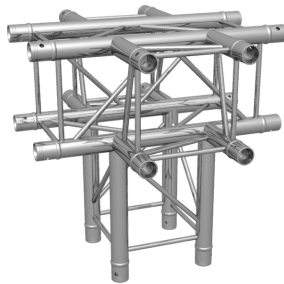
F24 5-Wege Ecke F24 5-way corner
