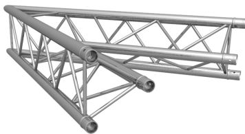
F23 2-Wege Ecke 45° innen F23 2-way corner 45° inside
