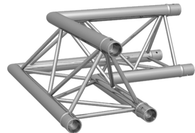
F23 2-Wege Ecke 90° F23 2-way corner 90°
