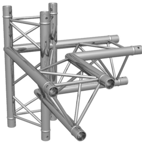
F23 4-Wege Ecke oben/links F23 4-way corner top/left
