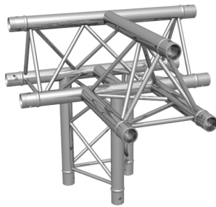
F23 4-Wege T-Stück oben F23 4-way T-piece top
