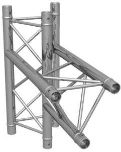
F23 3-Wege T-Stück vertikal F23 3-way T-piece vertical
