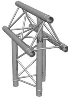
F23 3-Wege T-Stück horizontal F23 3-way T-piece horizontal
