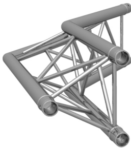
F23 2-Wege Ecke 135° außen F23 2-way corner 135° outside
