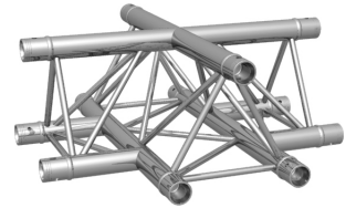
F23 4-Wege Kreuz F23 4-way cross
