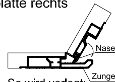
Normplatte (weisse/grau Ecken) = Mittelplatte oder Randplatte rechts
